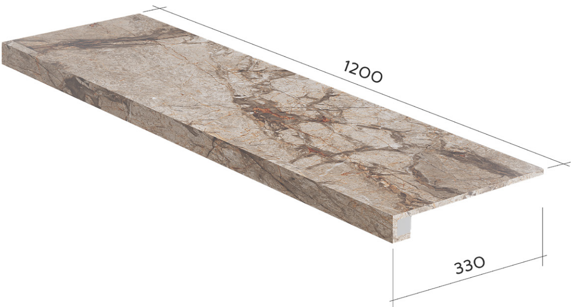
3D - модель
