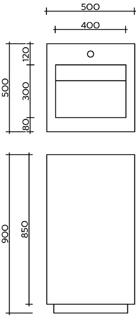
Чертеж
